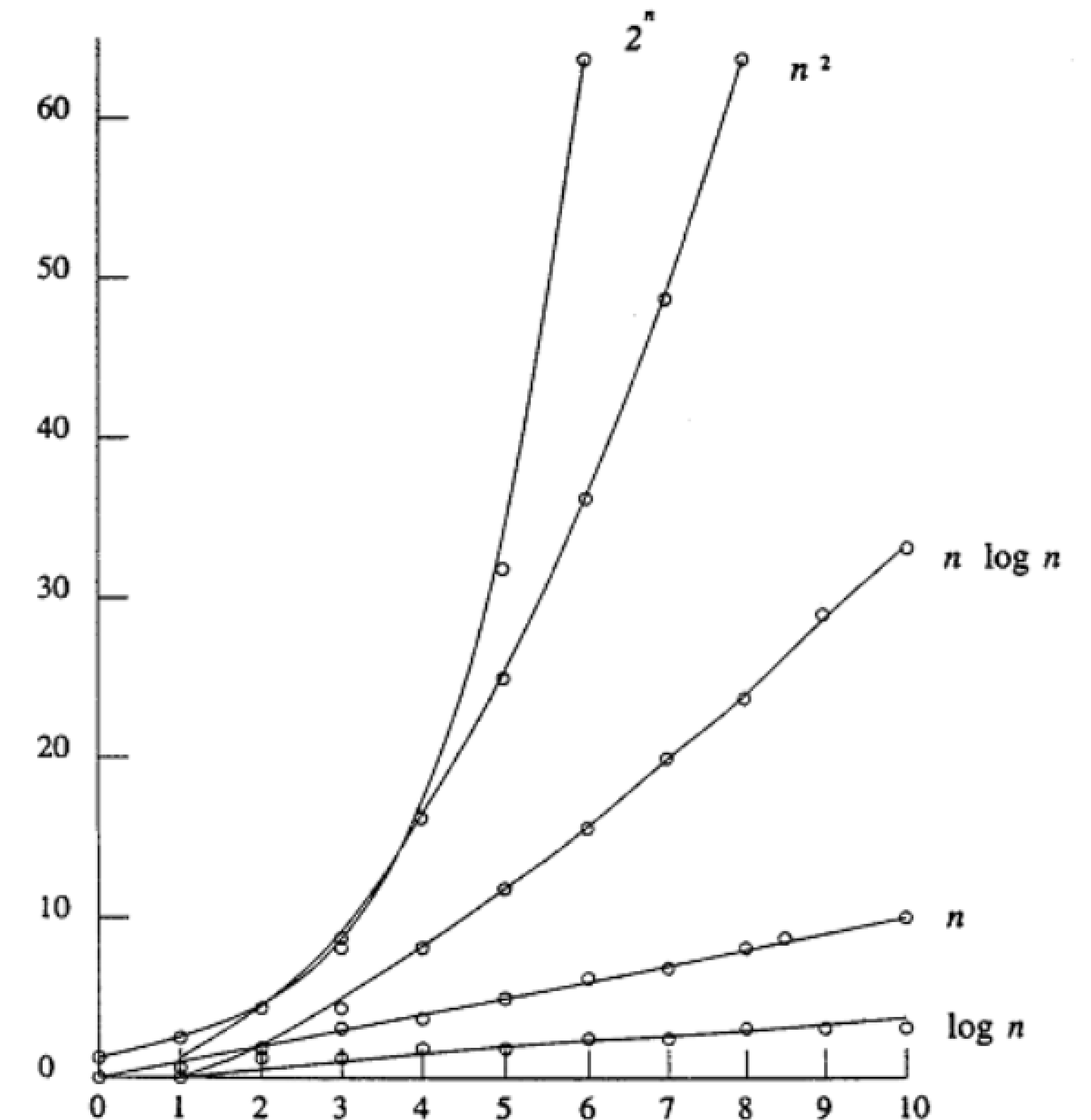
图2-1 时间复杂度函数曲线 blog.csdn.net/qq_41856733
